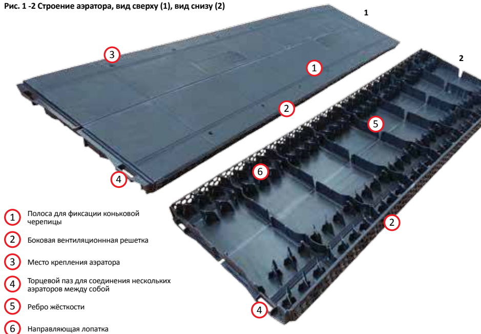
Рис. 1 -2 Строение аэратора, вид сверху (1), вид снизу (2)
